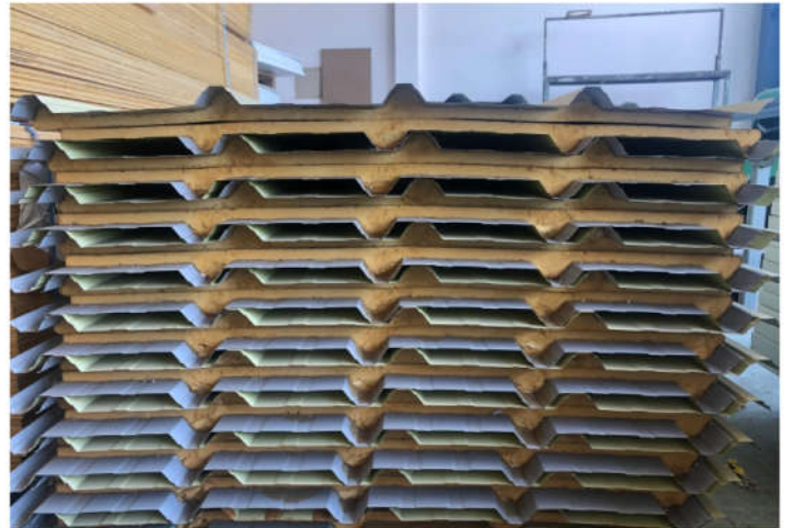
Mái sử dụng tôn cách nhiệt PU 断熱材PUの屋根
